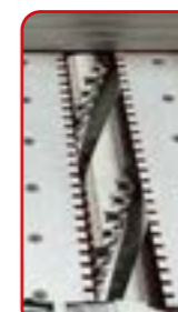
präzisionsgelagerte Spiral-Messerhobelwelle mit Wendeschneidplatten (4 Rillen a 17 Stück) precisely bedded spiral cutter block with in total 68 cutter inserts (4 grooves a 17 cutter inserts)
