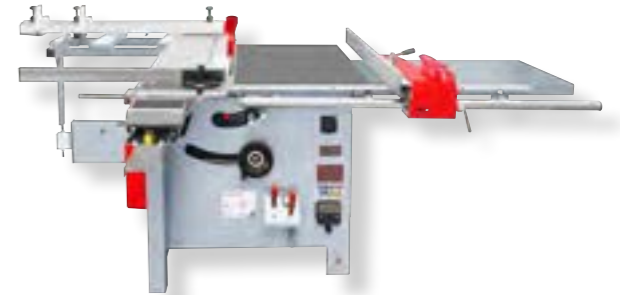
inklusive Vorritzer mit eigenem Motor und manueller Höhen und Seiteneinstellung including scorer with own motor and manual height and side adjustment
